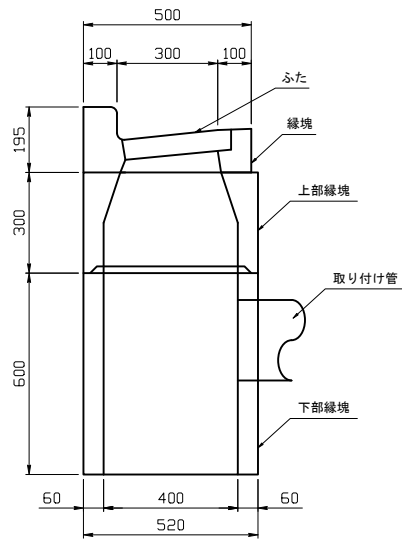
組立図
