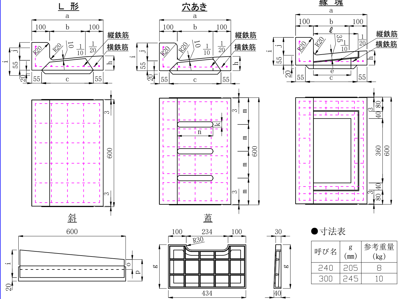
●寸法表
