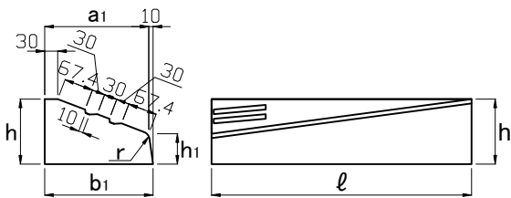
街渠 105型(斜1本使10cm落)
