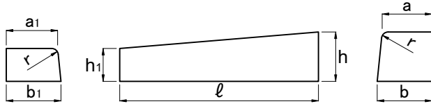
街渠 105型(斜1本使10cm落)
