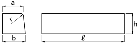
街渠 105型(都型車乗入れすりつけ左右)
