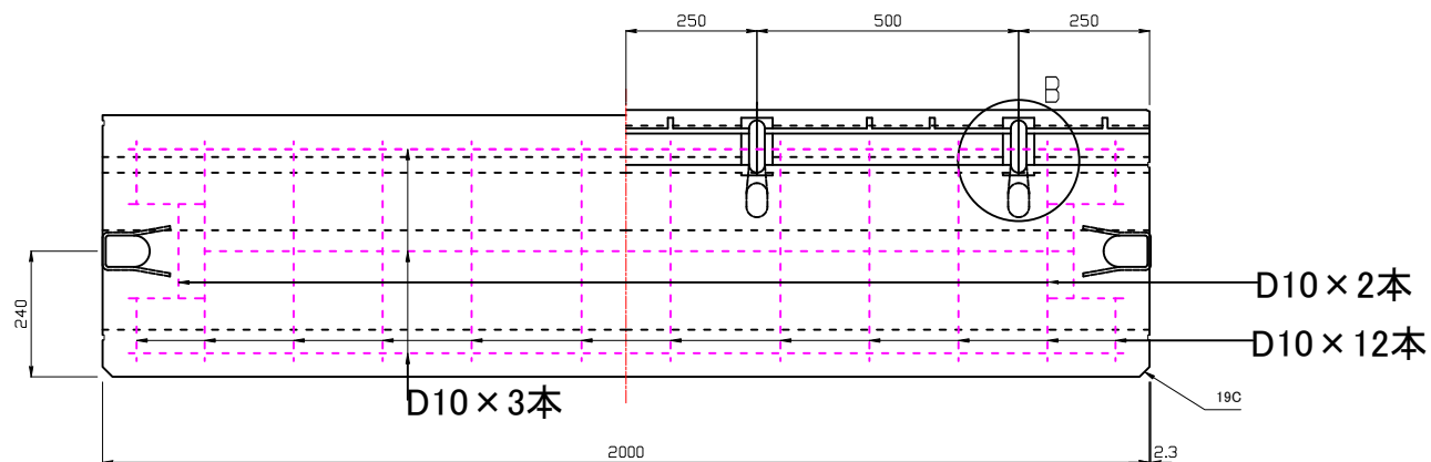
A-A面
